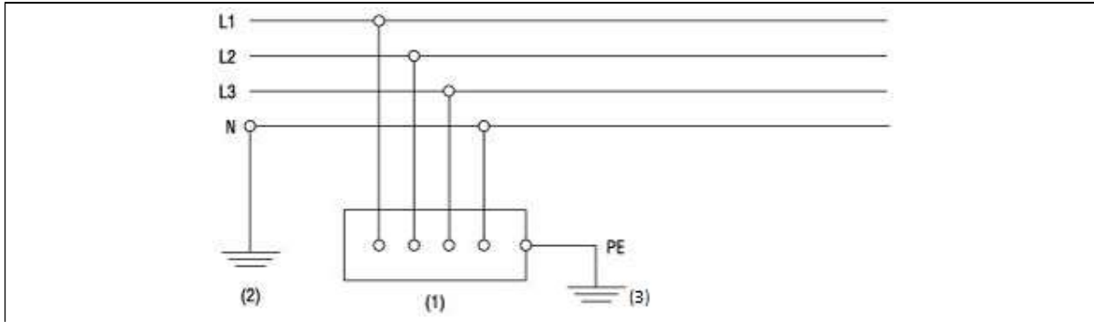
Figuur 3.4. TT-net
