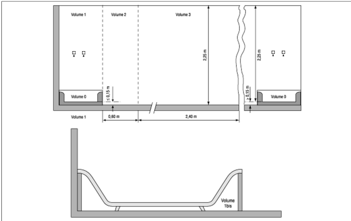
Figuur 7.11. Stortbadkuip – Vooraanzicht
