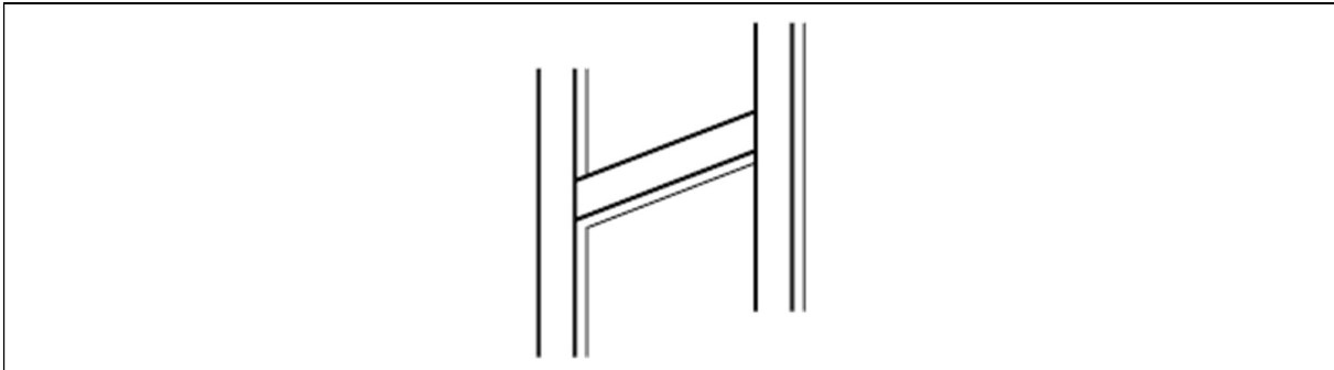
Figuur 5.21. Plaatsingswijzen van elektrische leidingen – Achter wandpanelen
