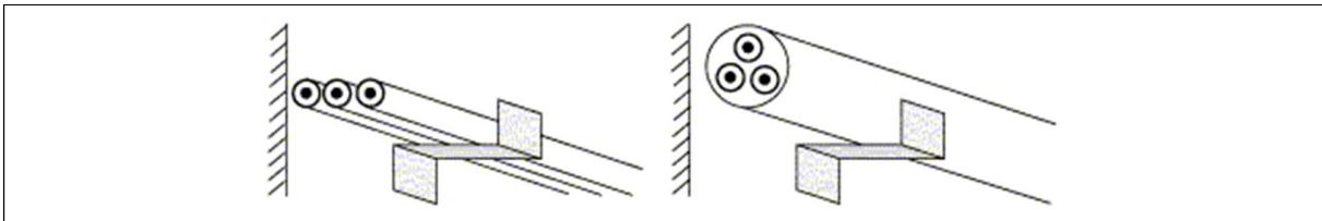
Figuur 5.10. Plaatsingswijzen van elektrische leidingen – Haken
