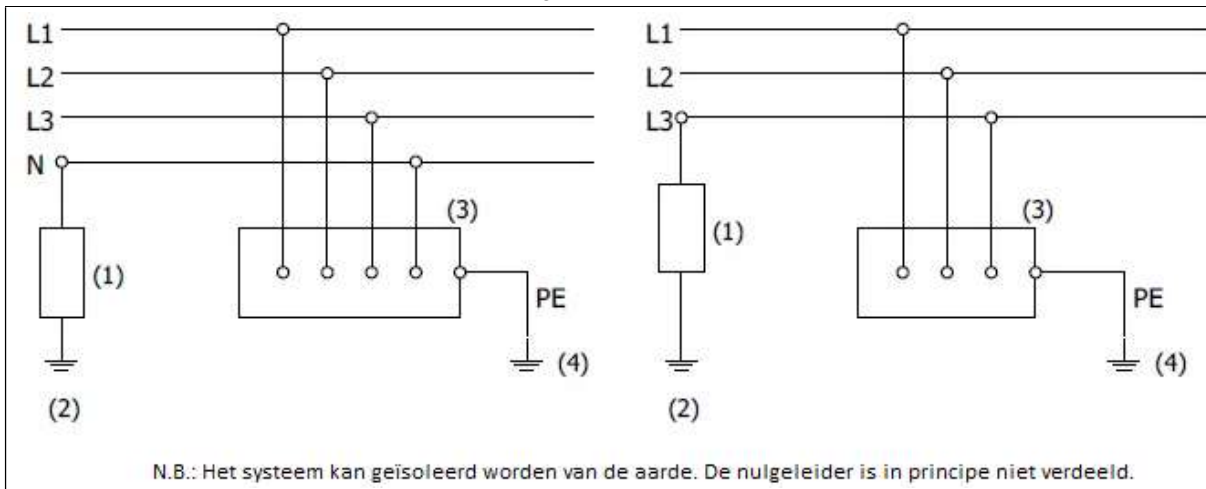
Figuur 3.5. IT-net
