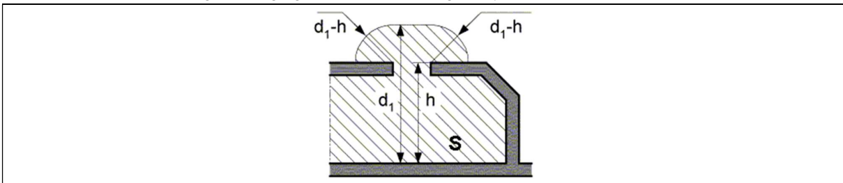
Figuur 2.9. Genaakbaarheidsgabariet: materiële elementen die het verplaatsingsoppervlak begrenzen hebben openingen die geen doorgang verlenen aan een lange staaf van 12 mm diameter
