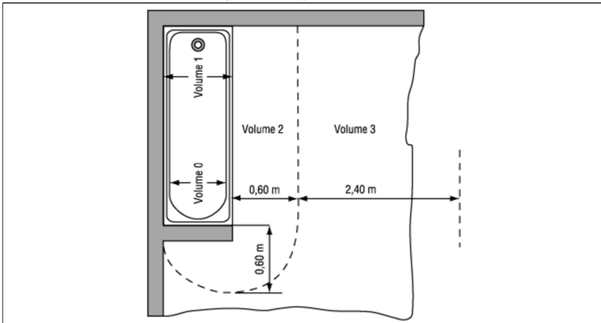
Figuur 7.2. Badkuip met vaste wand
