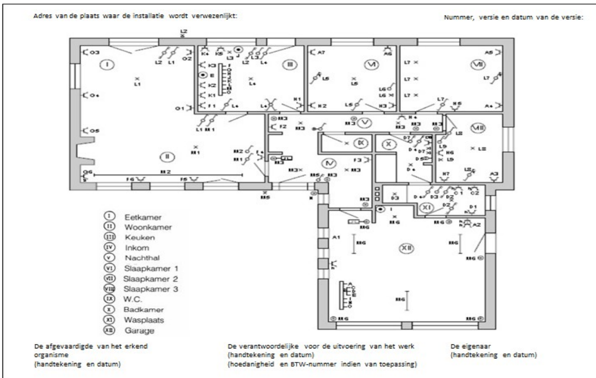
Figuur 3.2. Voorbeeld van een situatieplan
