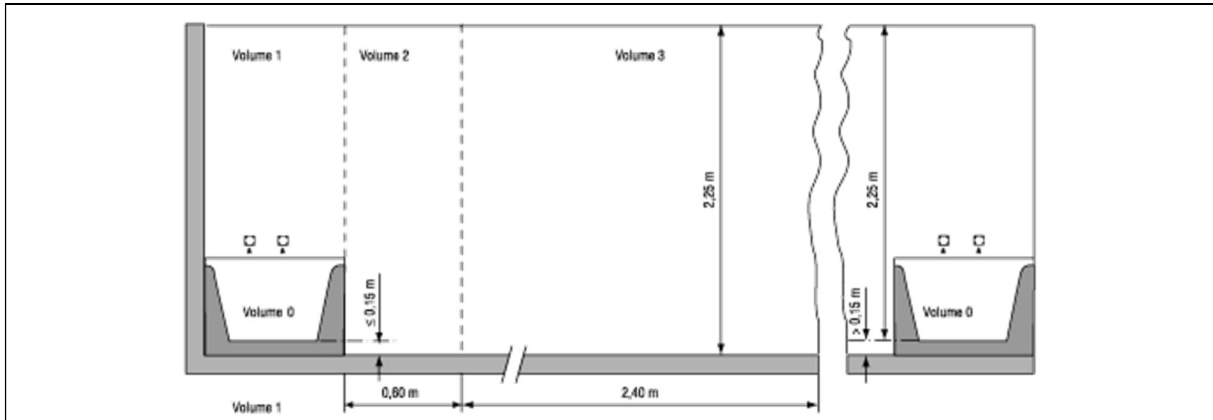
Figuur 7.10. Badkuip – Vooraanzicht
