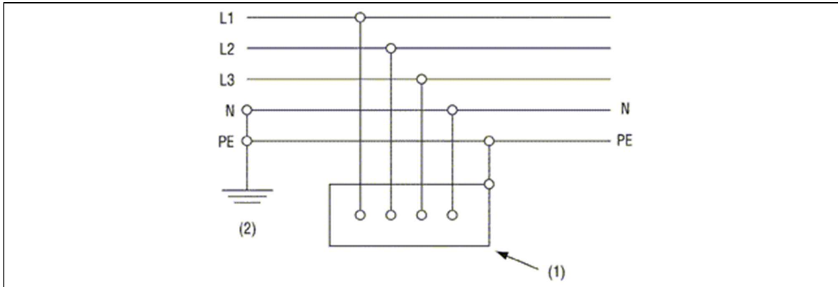
Figuur 2.1. TN-S-systeem
