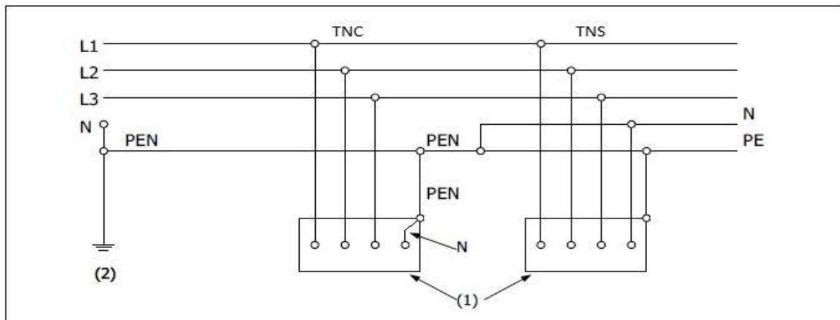
Figuur 3.3. TN-C-S-net
