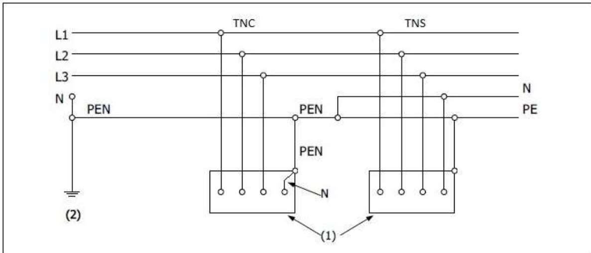
Figuur 2.3. TN-C-S-systeem
