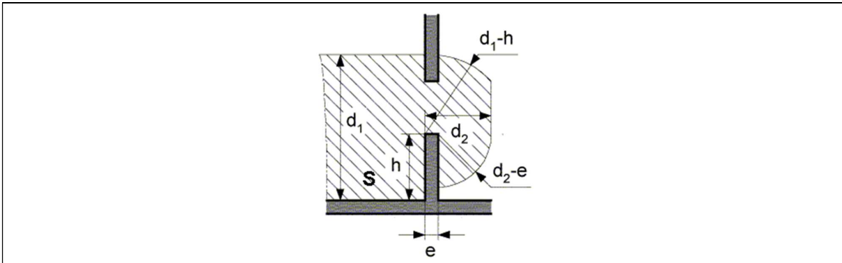
Figuur 2.9. Genaakbaarheidsgabariet: materiële elementen die het verplaatsingsoppervlak begrenzen hebben openingen die geen doorgang verlenen aan een lange staaf van 12 mm diameter
