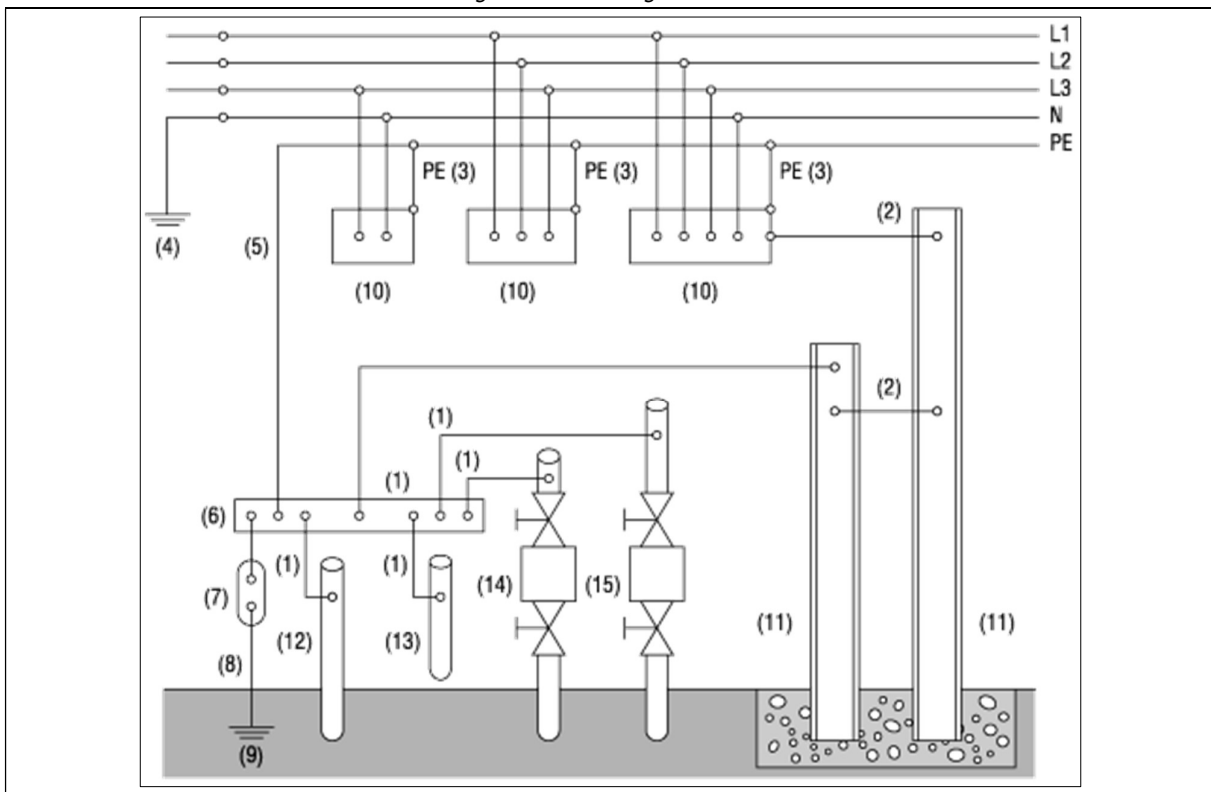
Figuur 2.10. Aardingsinstallatie
