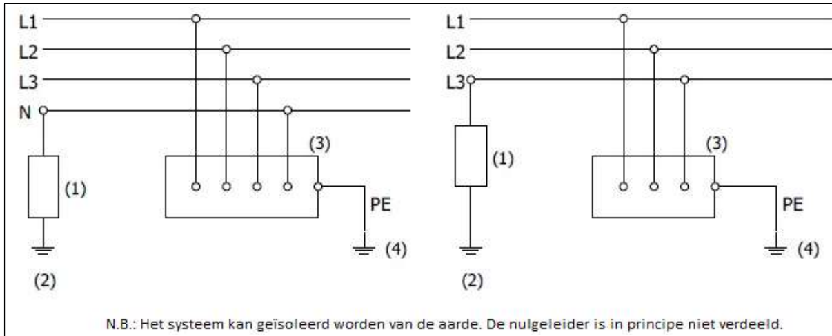
Figuur 2.5. IT-systeem
