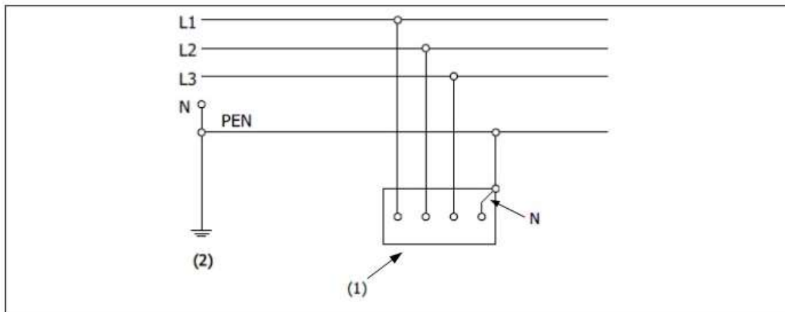
Figuur 2.2. TN-C-systeem
