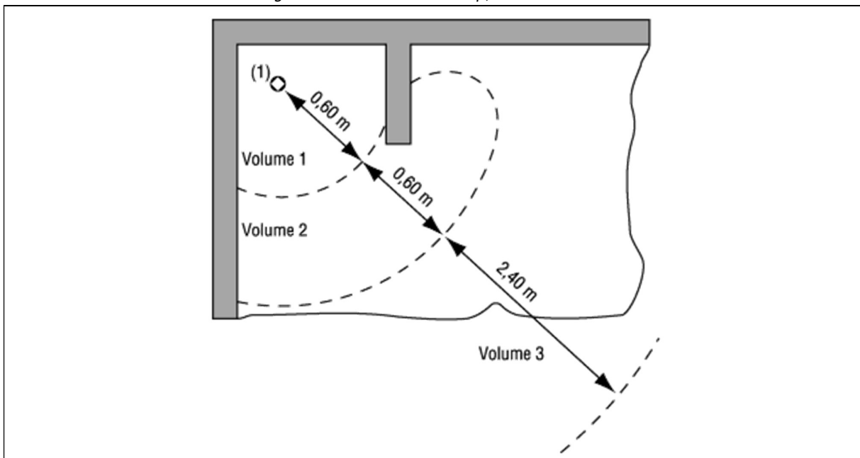
Figuur 7.6. Stortbad zonder kuip, met vaste wand
