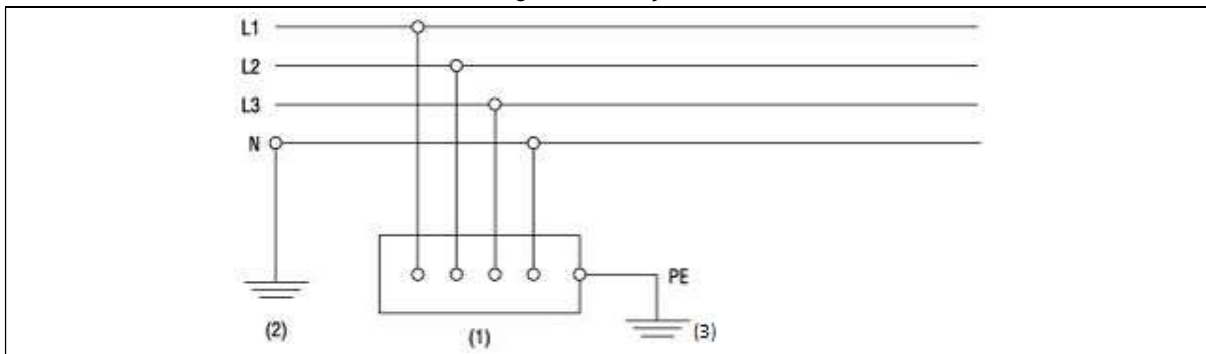
Figuur 2.4. TT-systeem
