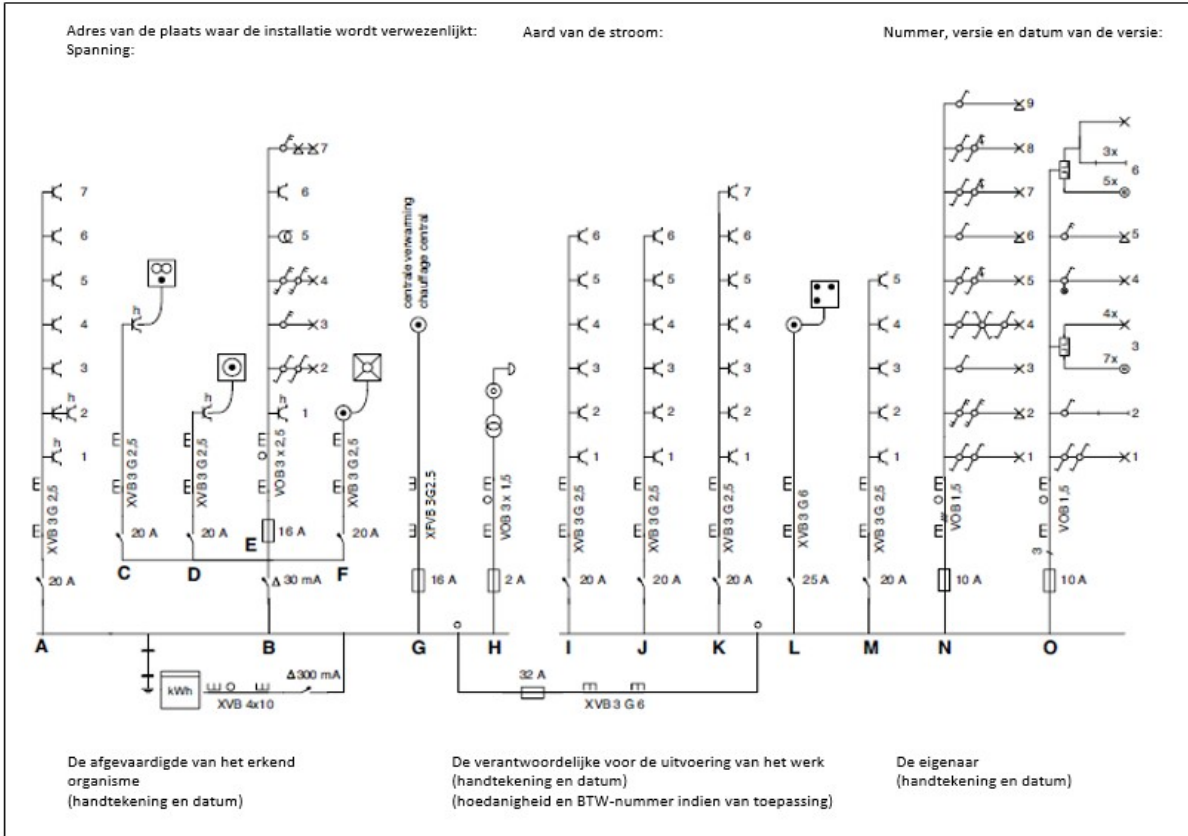
Figuur 3.1. Voorbeeld van een eendraadsschema
