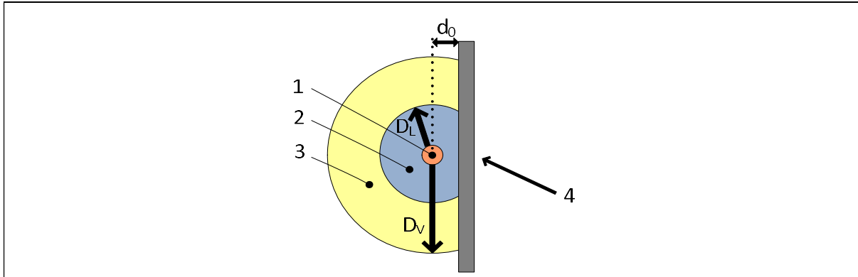
Figuur 2.23. Voorstelling van de zone onder spanning en de nabijheidszone met geaarde, metalen beschermrichting
