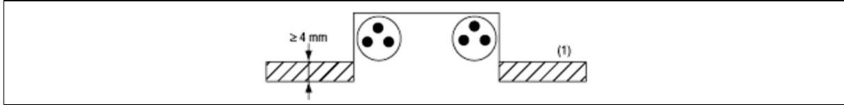
Figuur 5.28. Schematische doorsnede van een sleuf
